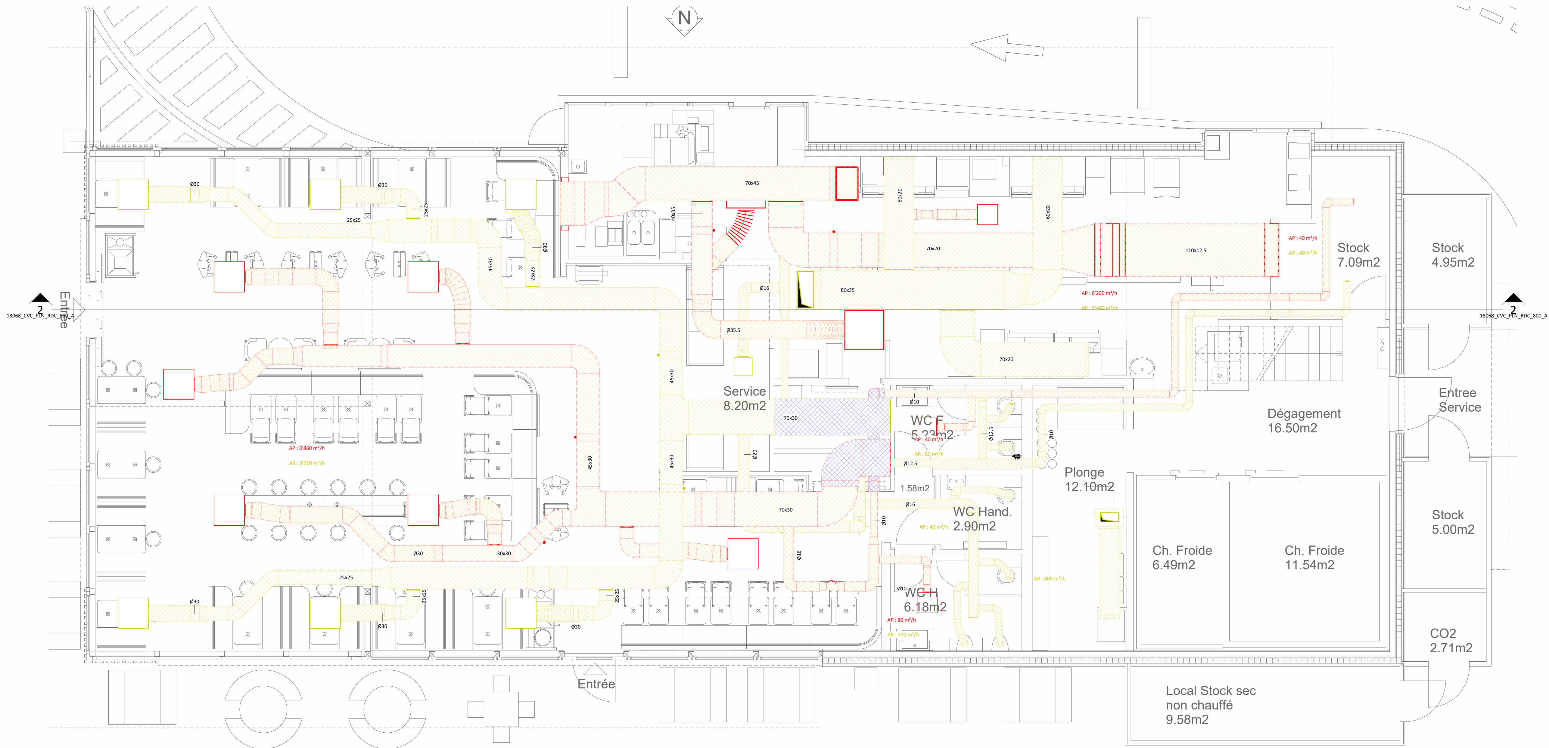
① RDC_CVC Soumission 1 : 50
