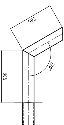
Detail Pos. 6 / detail pos. 6
