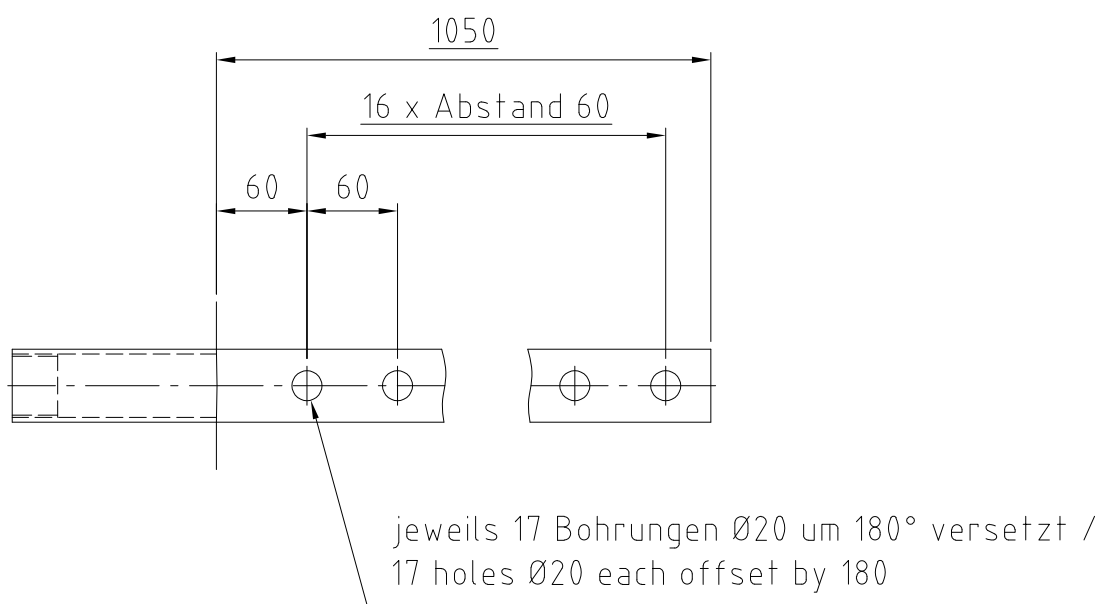
Detail Pos. 5 / detail pos. 5
