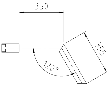
Detail Pos. 2 u. 6 / detail pos. 2 and 6
