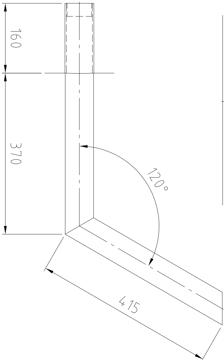
Detail Pos. 3-6 / detail pos. 3-6
