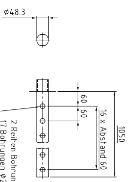
Detail Sprührohr Pos. 4 / detail spray tube pos.4
