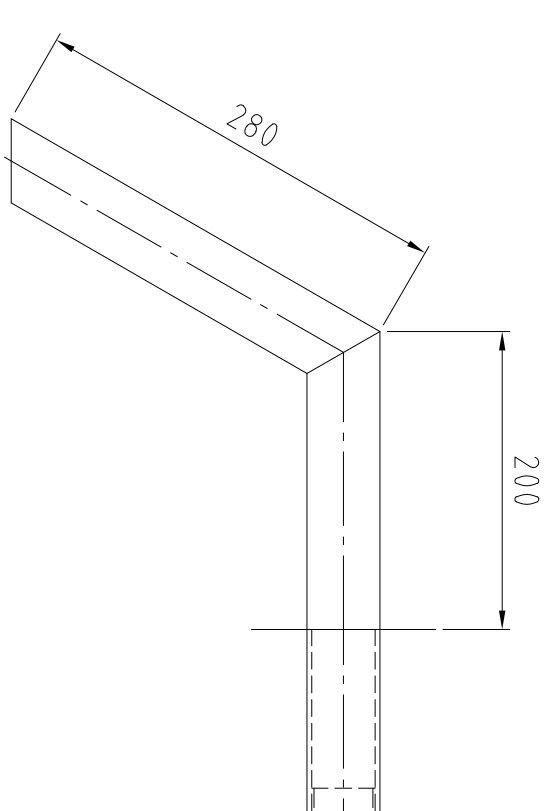
Detail Pos. 6, 9, 12 und 13
